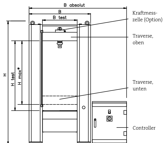
Vorderansicht Prüfmaschine mit Hauptabmessungen
