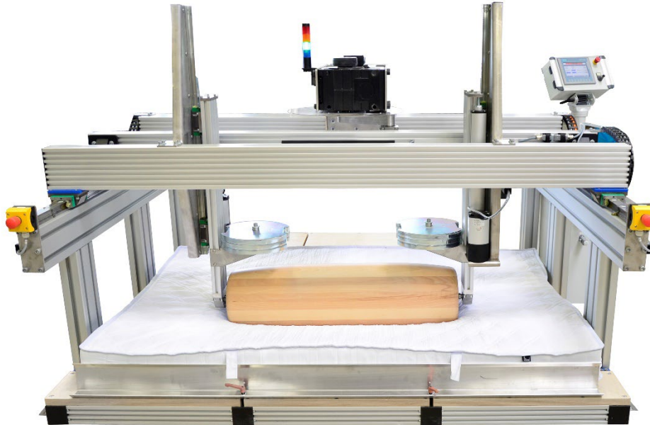
Einzelprüfstand für die Dauerhaltbarkeit von Matratzen, Federkernen und (Boxspring-)Betten nach EN 1957 (Art.-Nr.: 40-830-164)
