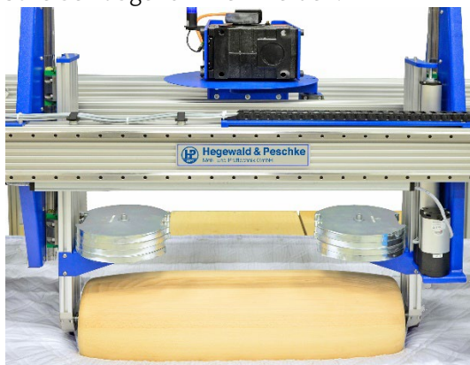
Belastungseinrichtung mit Gewichtsscheiben
