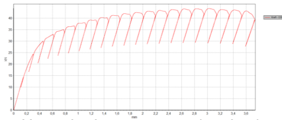
Abb.3: Teilentlastungen im Kraft-Kerbaufweitung-Diagramm
