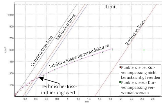
Abb.5: Risswiderstandskurve
