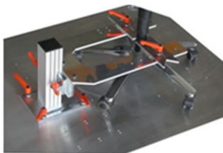
40-001-115 Universelle Haltevorrichtung für Fußkreuze von Sitzmöbeln ; höhenverstellbar
